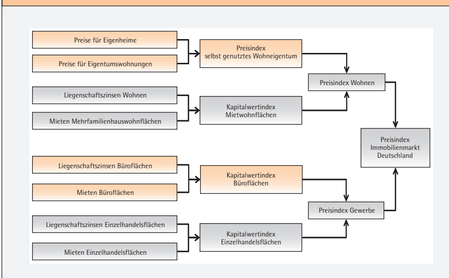
Abbildung 3: vdp-Indexfamilie
